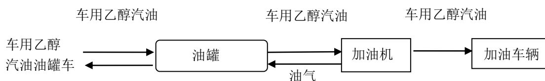
图2-4汽油加油及油气回收工艺流程图
