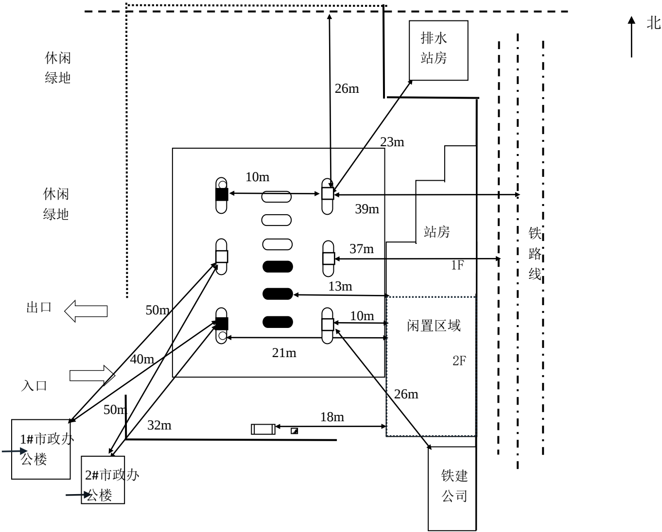
图 2-1 周边环境及总平面布置图
