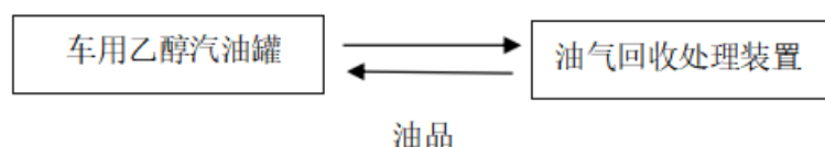
图 2-4 三次油气回收工艺流程图
