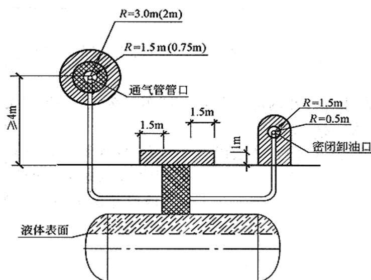
图 3-3 汽油埋地卧式储罐爆炸危险区域划分
