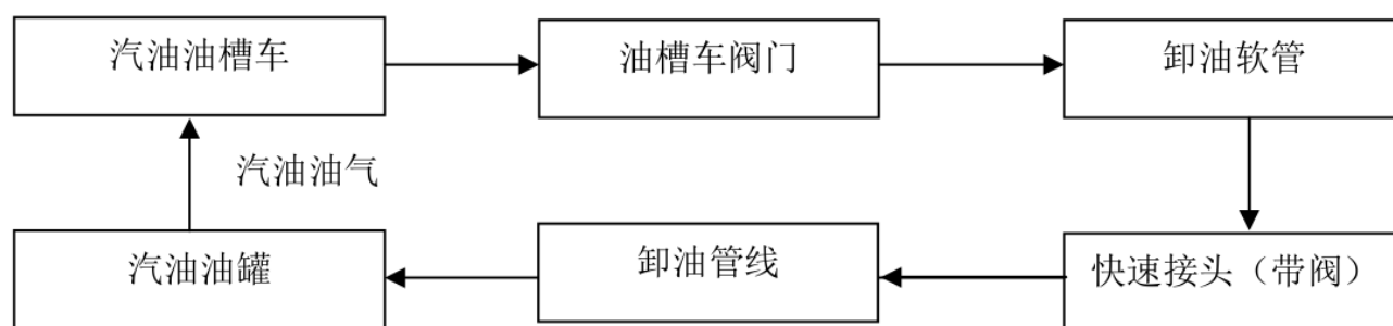
图 2-2 汽油卸油流程图
