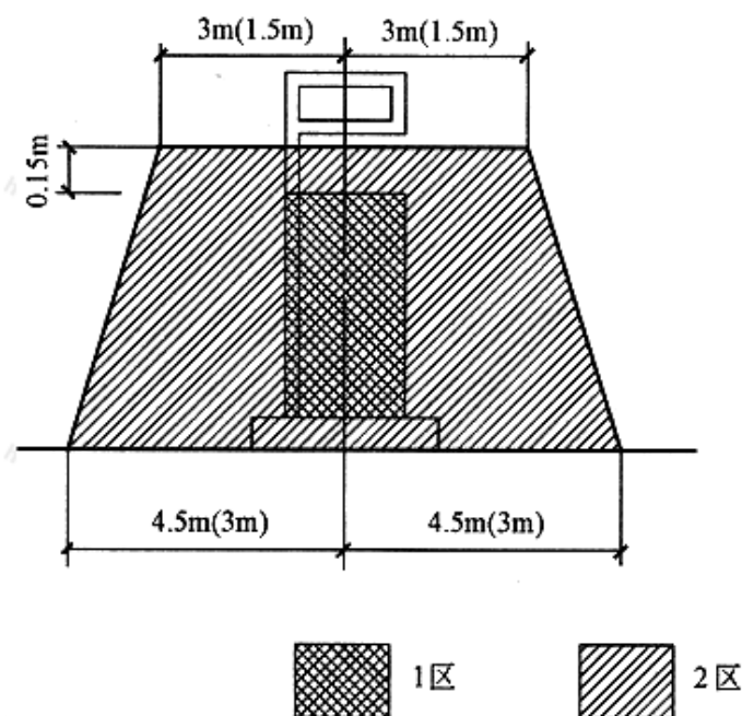
图 3-1 汽油加油机爆炸危险区域划分
