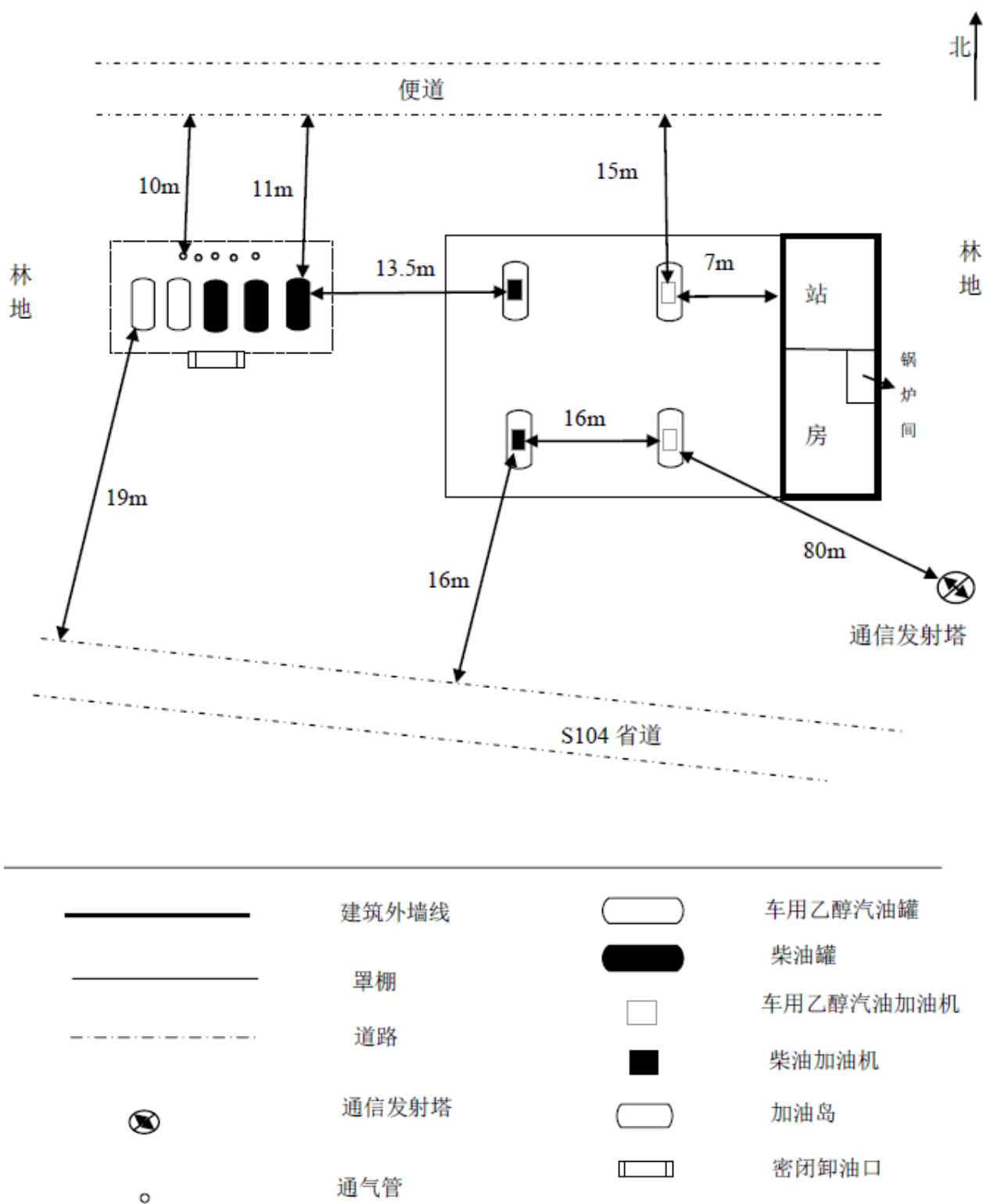
图 2-1 周边环境及总平面布置图
