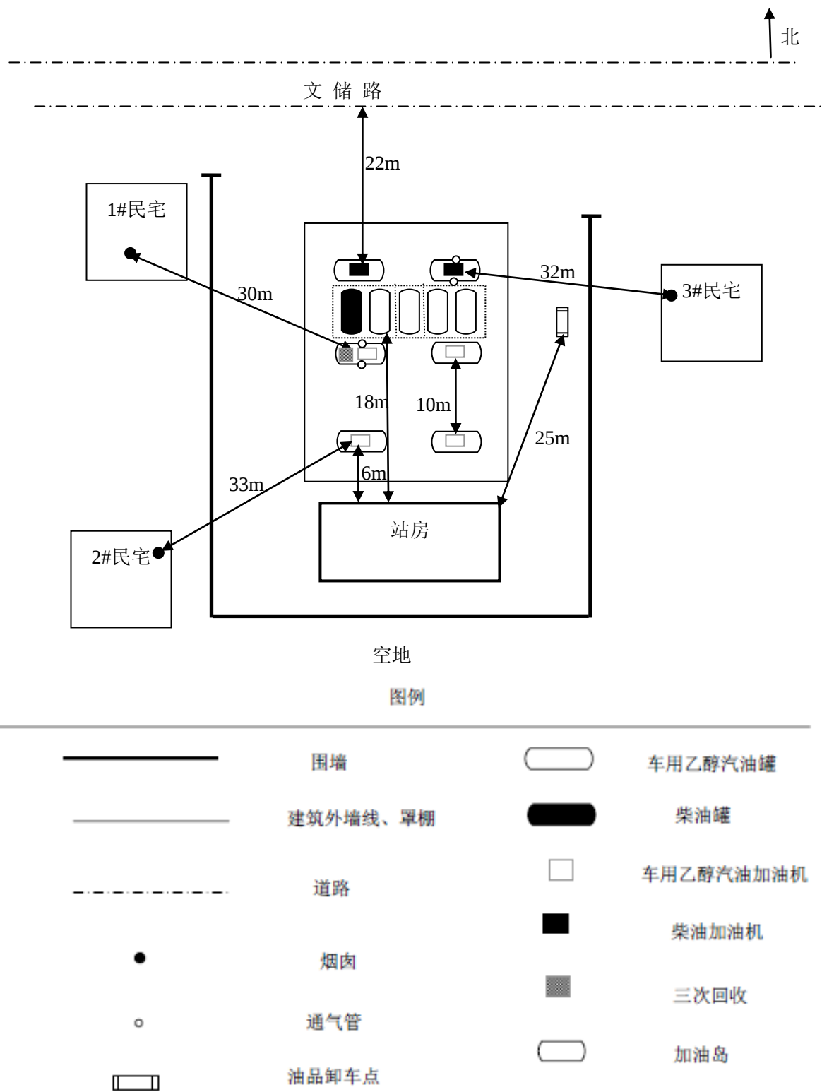
图 2-1 周边环境及总平面布置图
